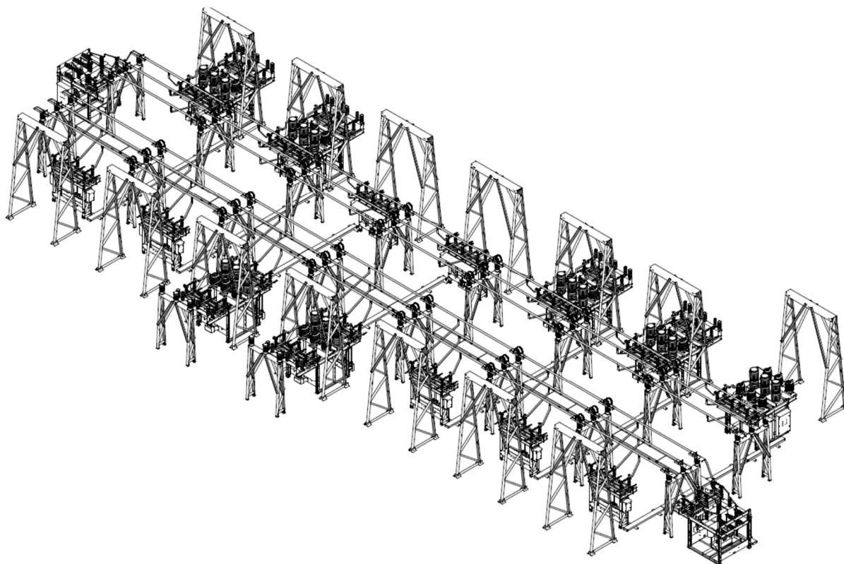
ОРУ-35 13 схема
